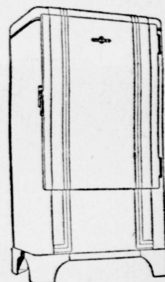
DRS Model
