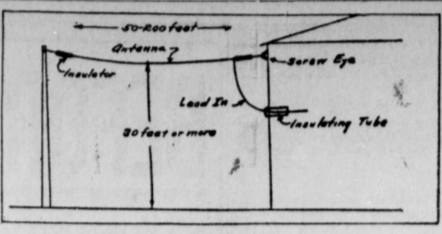
The Antenna.
